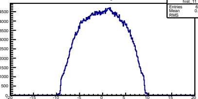
MID T left -T right [ns]
