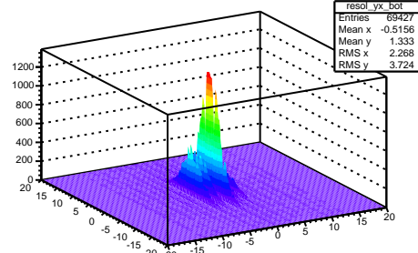
BOT Y vs X resolution
