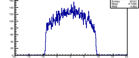
BOT T left -T right [ns]
