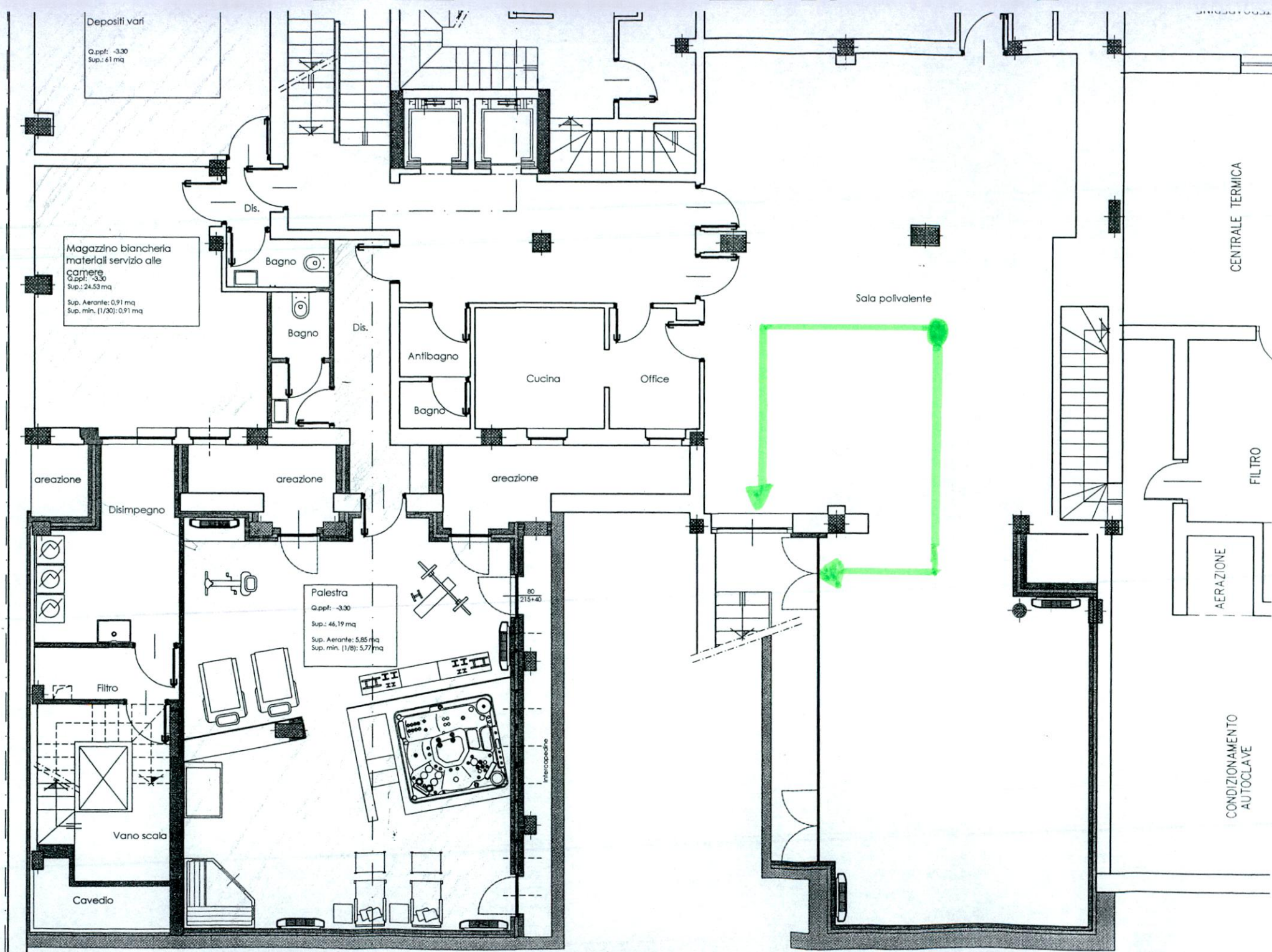
PIANTA PIANO PRIMO INTERRATO
